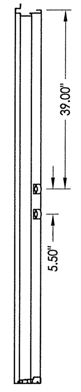
STRIKE JAMB
