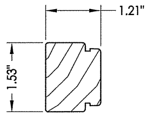
12 HINGE STILE
