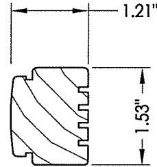
11 LATCH STILE
